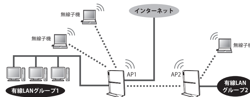
図1 無線APが4台の例
