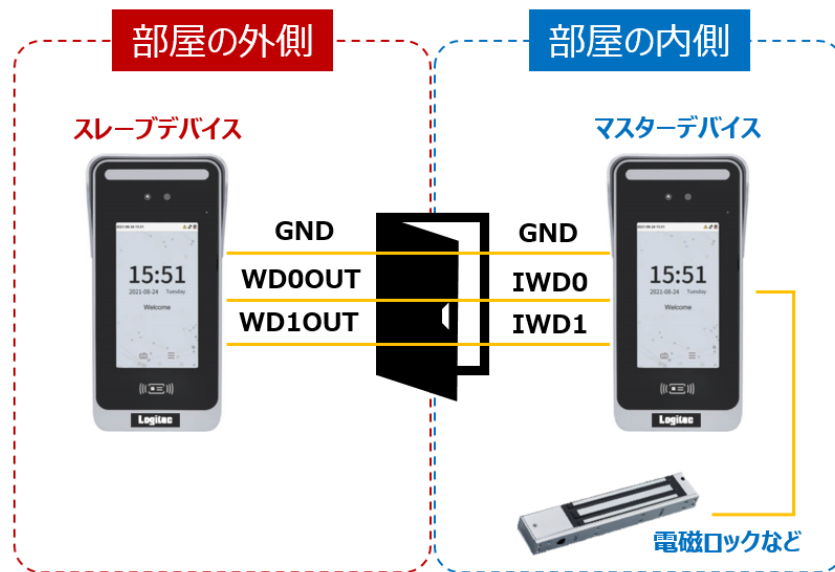
【配線図】
